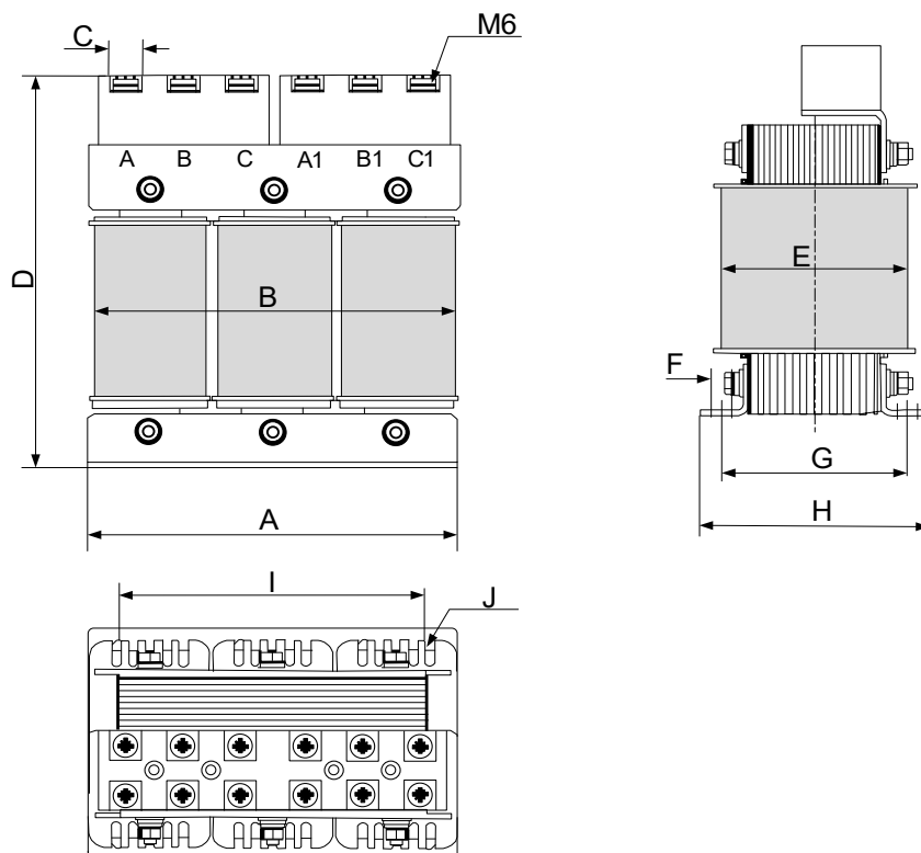
Рис. 8-2 Размеры входных реакторов переменного тока 40 А (1,45 мГн)
