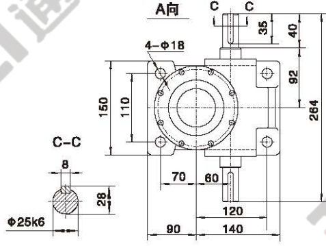
双输入 Double input shaft
