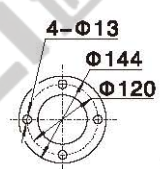
M型 /M shape
