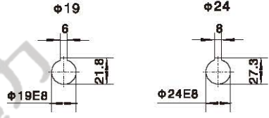
直联双输入 Direct double input shaft
