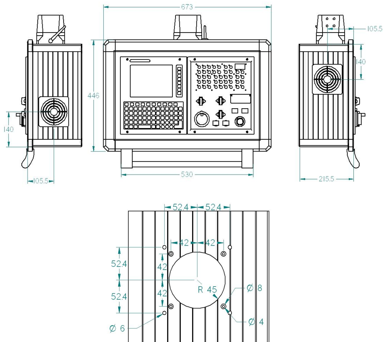
Схема расположения отверстий для крепежных винтов вентилятора
