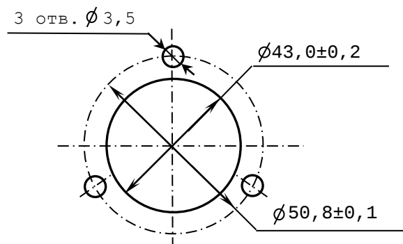
Рисунок Г.9 - Установочные размеры штурвала WSB
