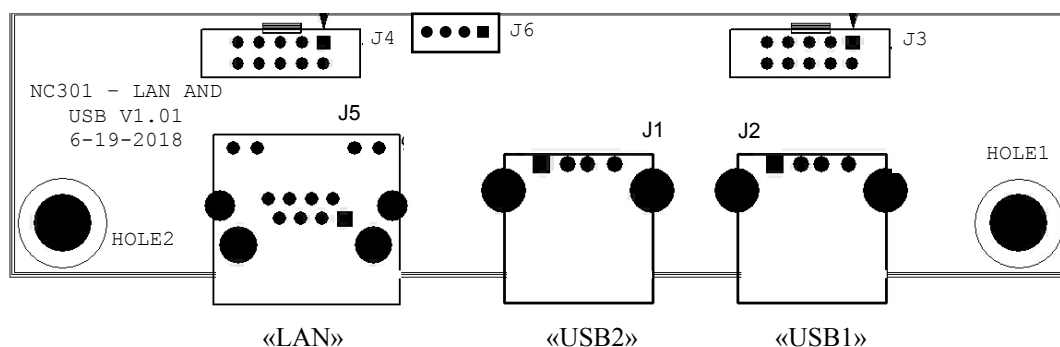
Рисунок 4.24 – Плата разъёмов LAN AND USB NC301-25 (V1.01)
