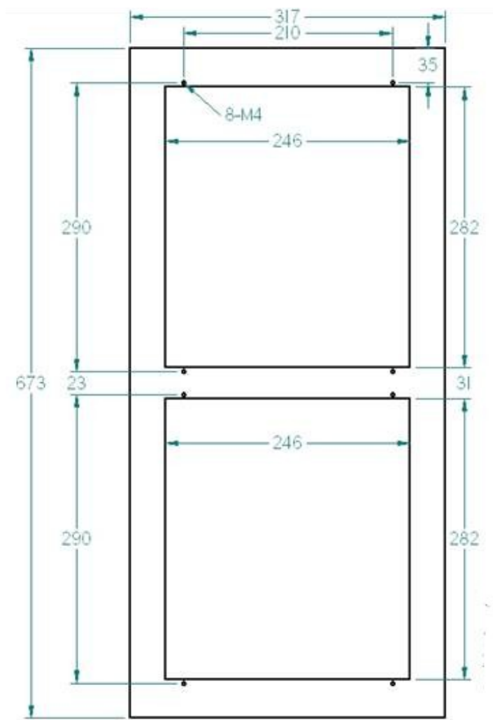
Рисунок Ж.5 – Размеры передней части лицевой панели кожуха вертикального типа для УЧПУ NC-301.
