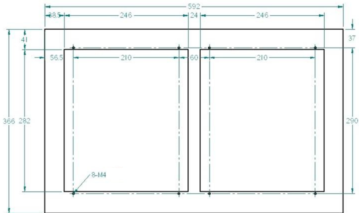
Рисунок Ж.6 – Размеры передней части лицевой панели кожуха горизонтального типа для УЧПУ NC-301.
