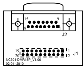
б) плата разъемов RS422 NC301-311
