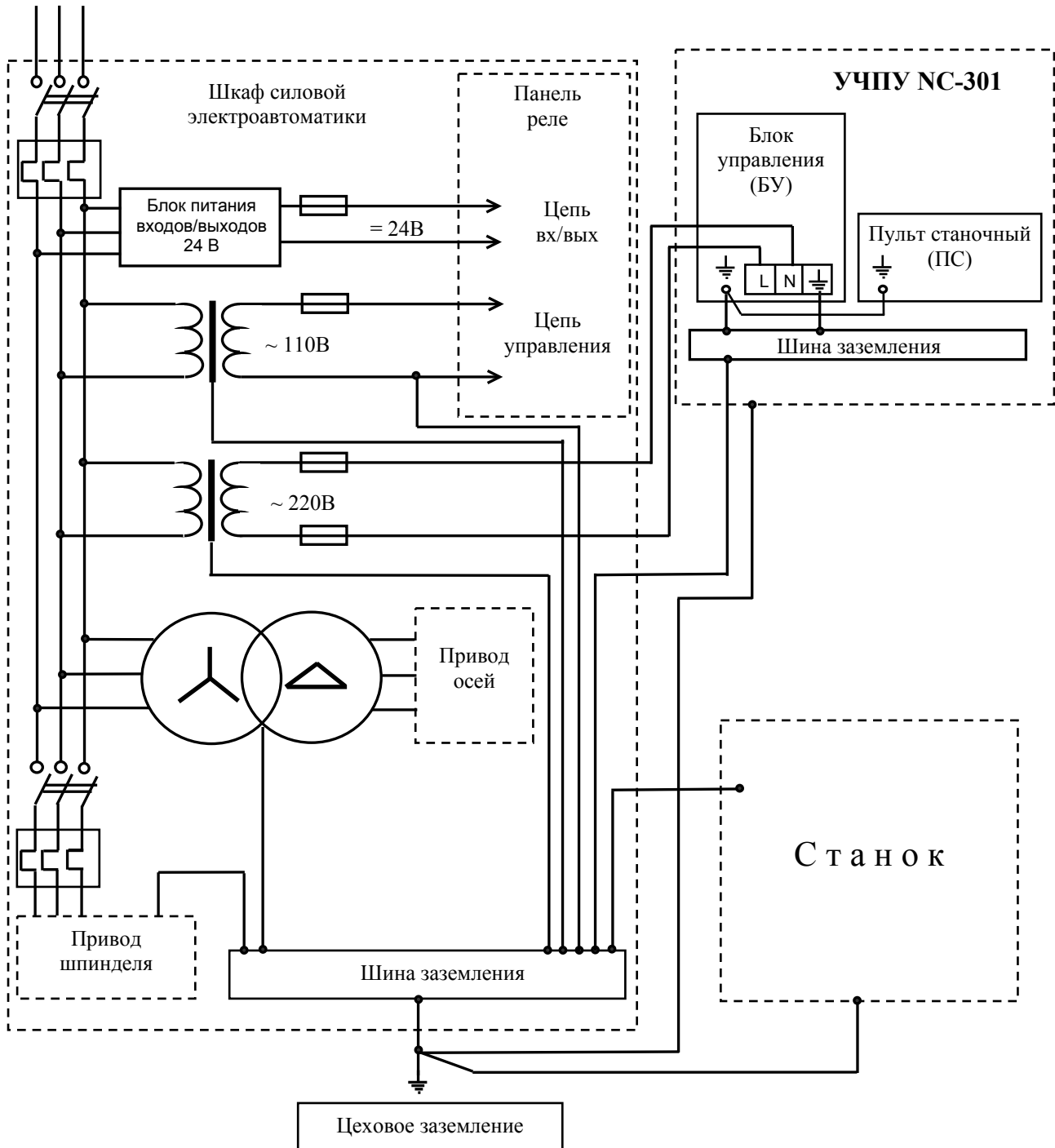
Рисунок 3.1 – Схема подключения УЧПУ NC-301
