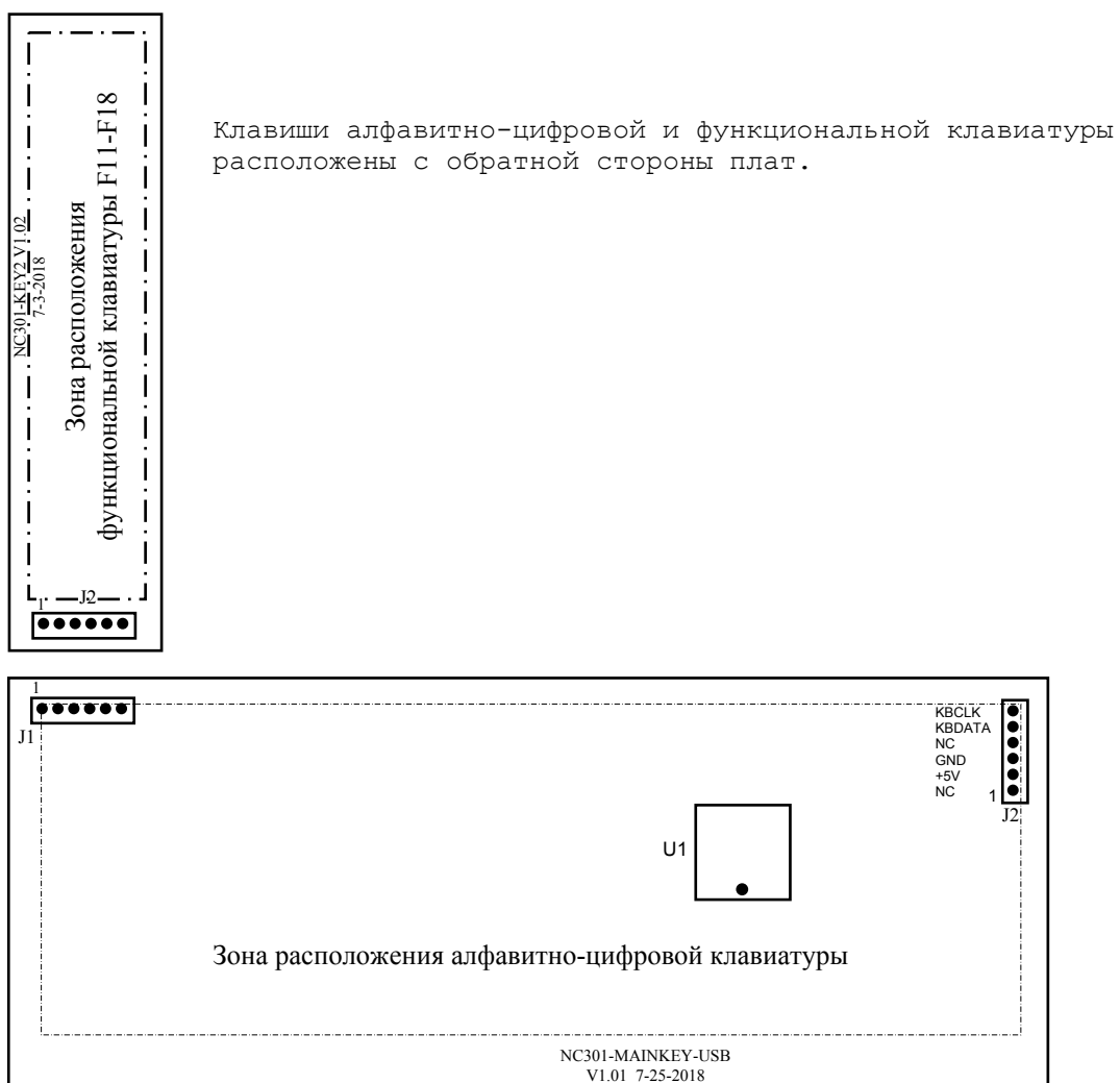
Рисунок 4.27 – Расположение разъемов плат NC301-29 и NC301-2A
