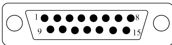
Рисунок 4.19 – Расположение контактов разъёма «C15-422» (вилка DPS 15-M)
