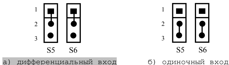
Рисунок 4.27 - Выбор входа канала штурвала
