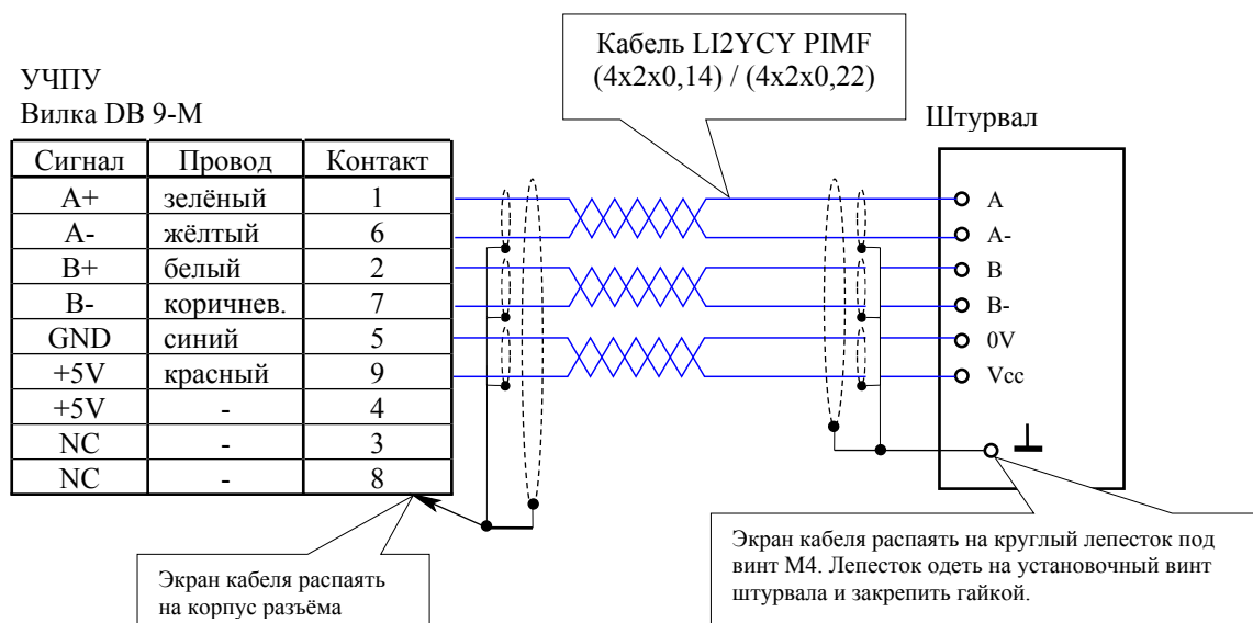
Рисунок В.6 – Схема кабеля штурвала
