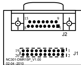
б) плата разъёмов RS422 NC301-311
