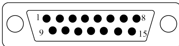
Рисунок 4.28 – Расположение контактов разъёма «C15-422»
