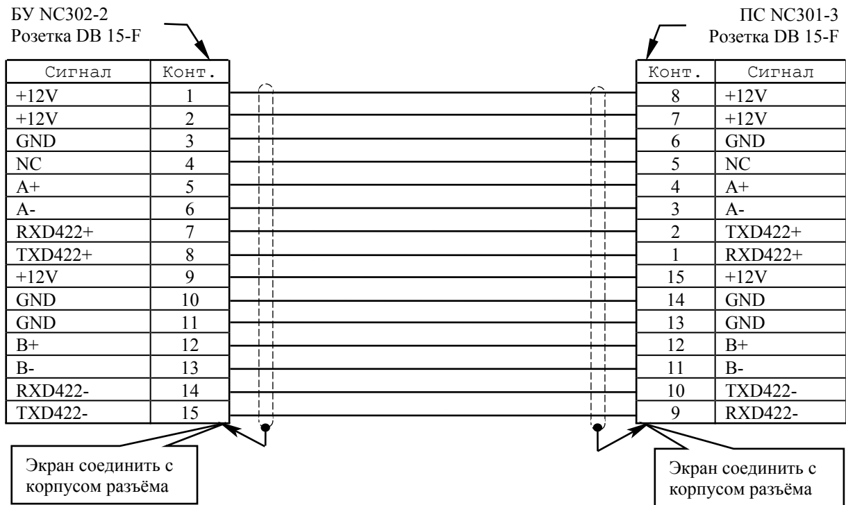
Рисунок 4.29 – Схема кабеля NC301-81
