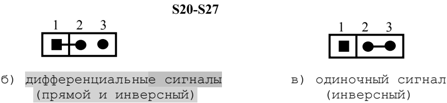
Рисунок 4.13 – Установка типа выходных сигналов канала ЦИП
