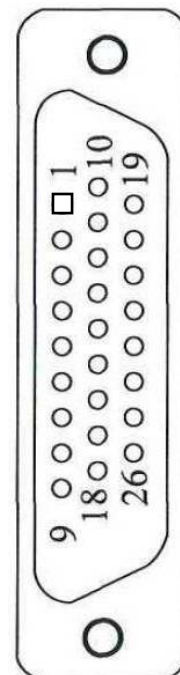
Рисунок 4.6 – разъем J2
