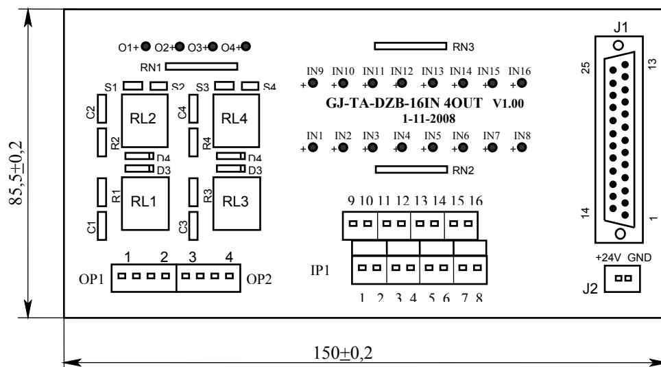
Рисунок Д.1 – Лицевая сторона платы модуля NC302-201
