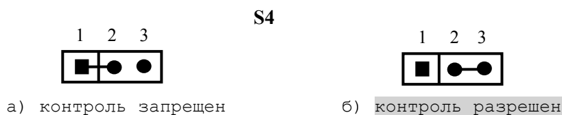
Рисунок 4.8 – Контроль обрыва сигналов энкодера
