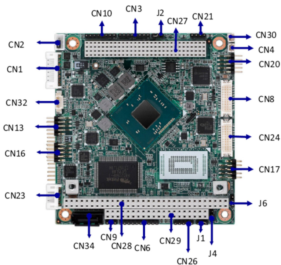
Верхняя сторона платы CPU PCM-3365
