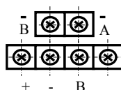
Рисунок 5.9 – Расположение выходных контактов штурвала ZBG-003-100
