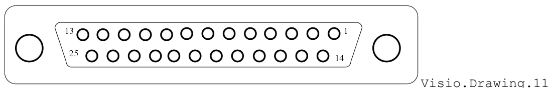
Рисунок 4.26 - Расположение контактов разъёма «I/O»
