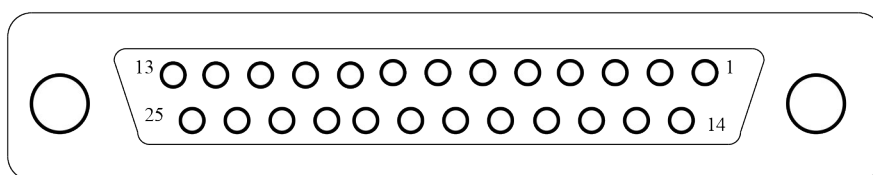
Сигналы разъема J11
