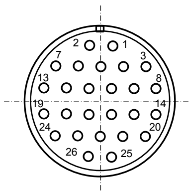
Рисунок Г.3 – Расположение контактов разъёма PCB NC110-78В
