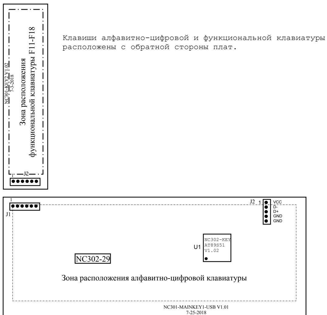
Рисунок 4.34 – Расположение разъёмов плат NC302-29 и NC302-2A
