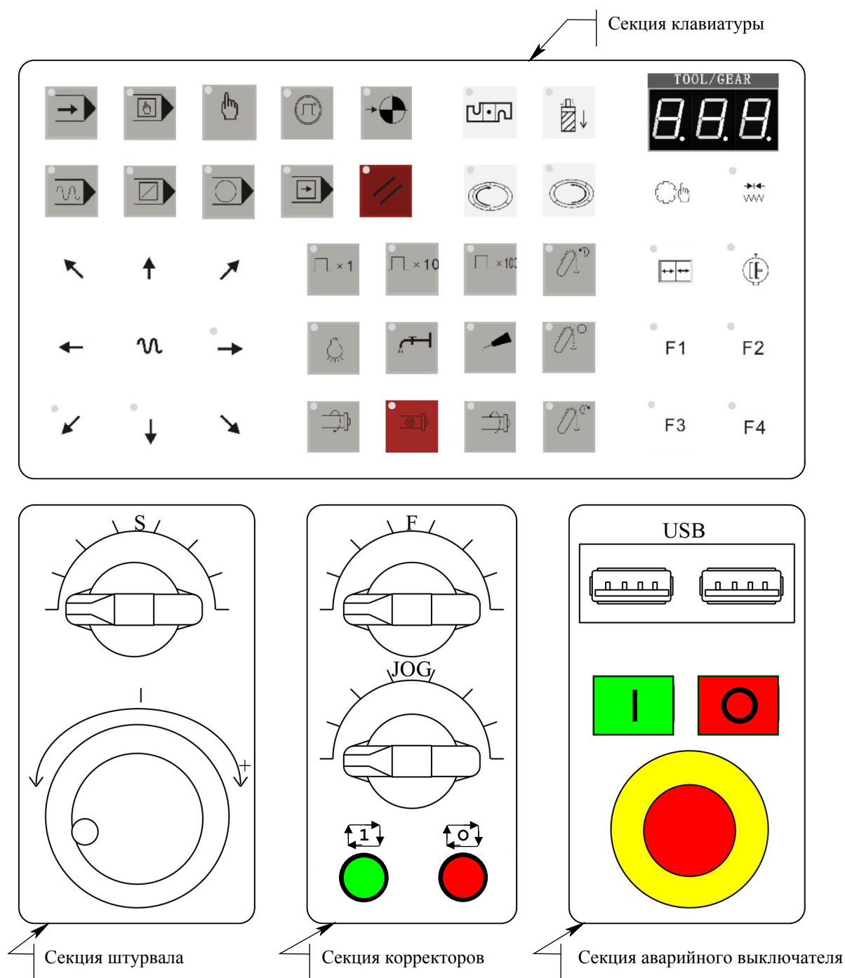
Рисунок 5.1 – Секции лицевой панели ПС NC301-3
