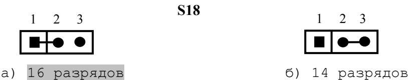
Рисунок 4.17 – Выбор разрядности ЦИП
