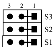
Рисунок 6.27 – Установка переключек джамперов S1-S3
