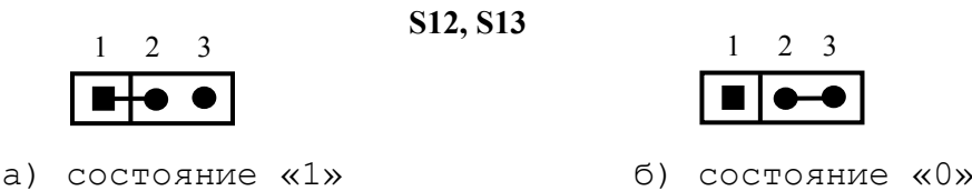
Рисунок 4.16 – Выбор дискретности ЦИП
