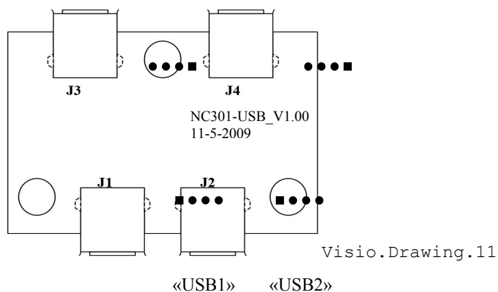
Рисунок 5.5 – Плата разъёмов USB NC301-33
