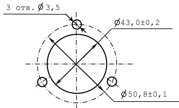
Рисунок Б.9 – Установочные размеры штурвала WSB
