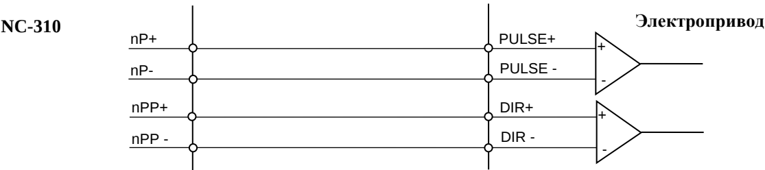
Рисунок 5.26 – Подключение дифференциальных сигналов ЦИП
