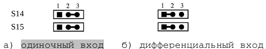
Рисунок 4.14 – Выбор входа электронного штурвала
