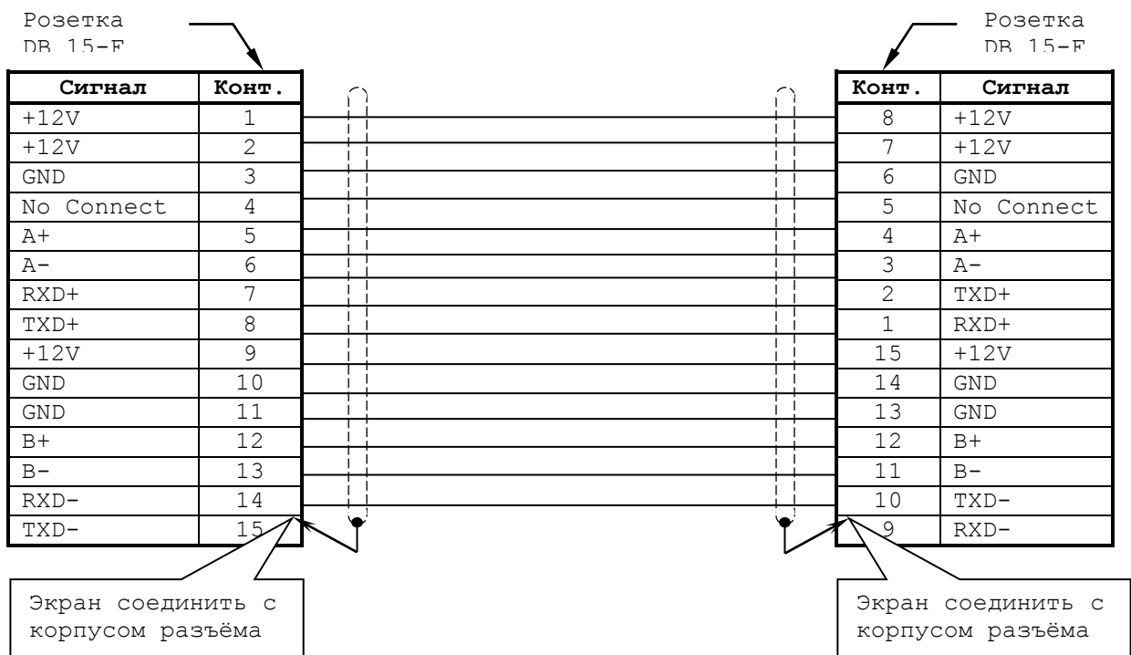
Рисунок 4.37 – Электрическая схема кабеля канала 422 NC310-82
