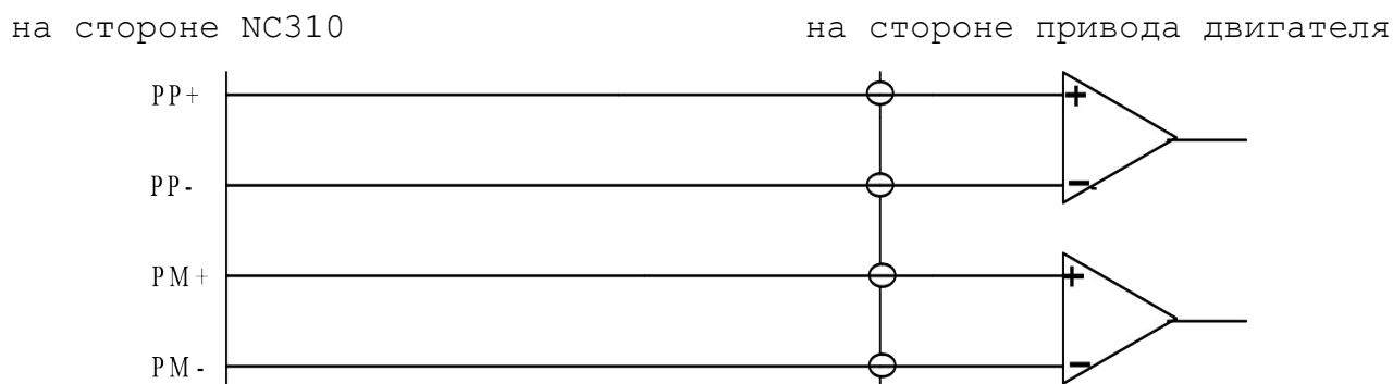
Рисунок 5.32 – Принципиальная схема подключения привода двигателя, который управляет входной линией приемника
