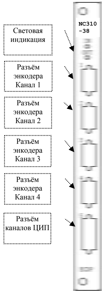
Рисунок 5.20 – Лицевая панель модуля ECDP
