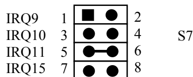
Рисунок 4.12 – Расположение контактов блока джамперов S7
