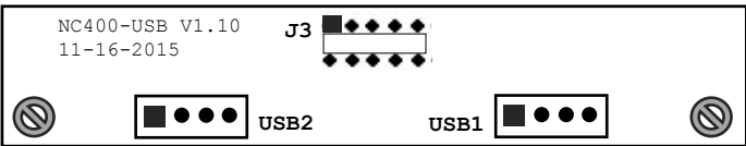
Рисунок 4.38 – Расположение разъёмов платы NC400-56
