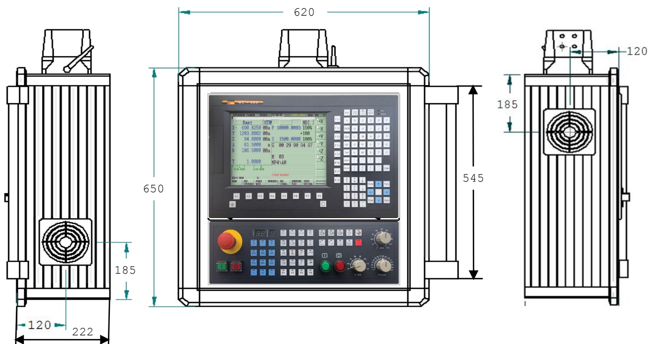
Рисунок Д.1 – Габаритные размеры кожуха для УЧПУ NC-400.
