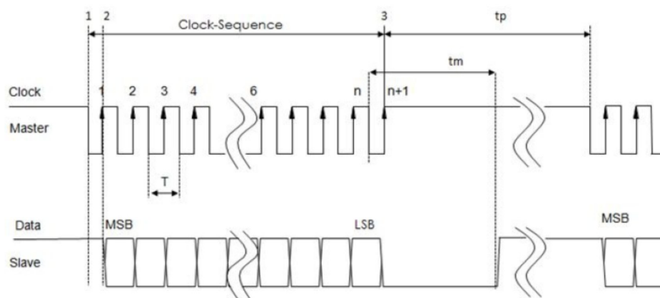
Диаграмма последовательности сигнала интерфейса SSI
