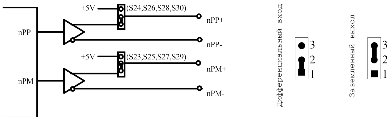
Рисунок 5.30 Структура выходов канала
