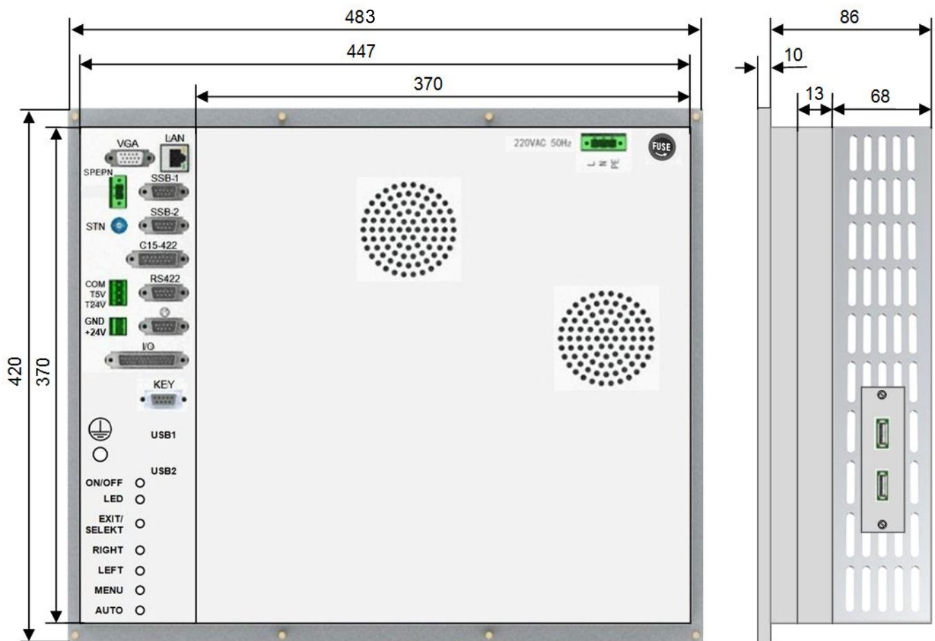
Рисунок 3.3 – Габаритные и установочные размеры блока управления NC400M-5
