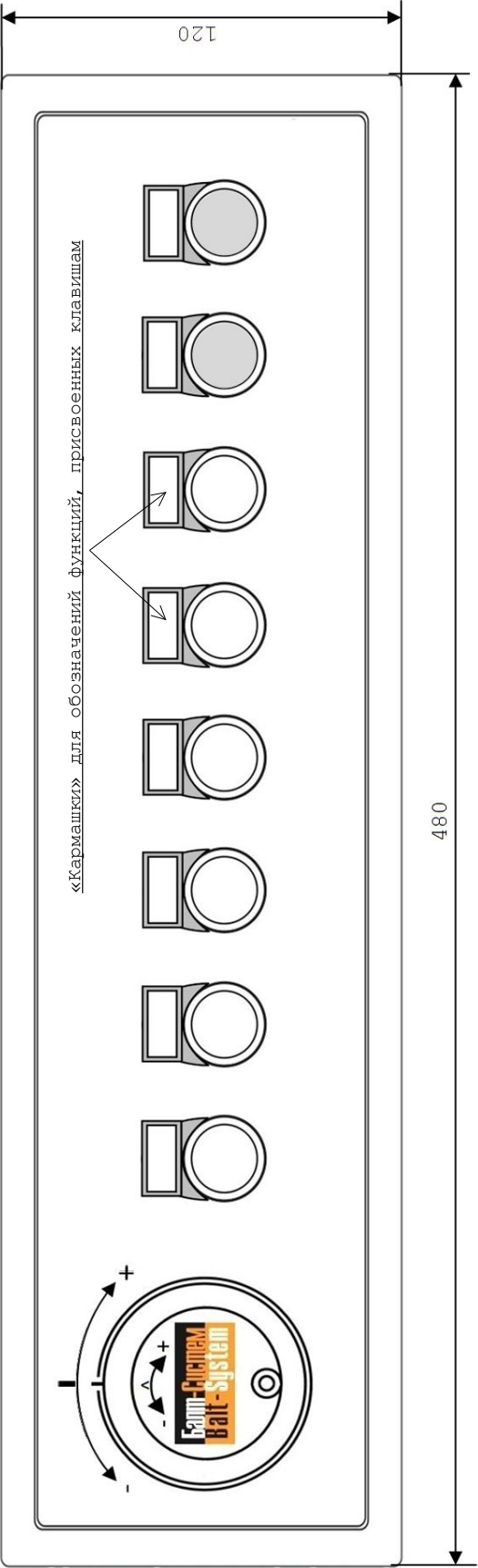
Рисунок 7.2 – Лицевая сторона дополнительной панели для управления станком NC400M-9
