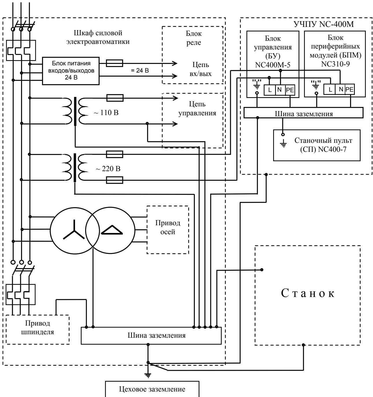
Рисунок Е.1 – Схема подключения УЧПУ NC-400М
