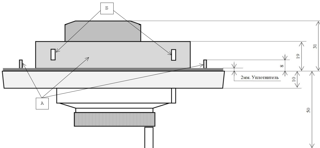
Рисунок 7.1 – Дополнительная панель для управления станком NC400М-9, вид сбоку.
