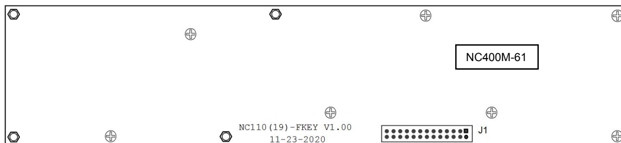
Рисунок 8.5 – Плата клавиатуры NC400M-61
