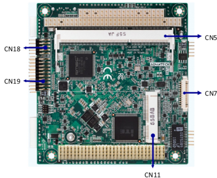
Нижняя сторона платы CPU PCM-3365
