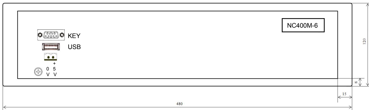
Рисунок 8.1 - Блок клавиатуры NC400М-6, корпус, вид сзади.
