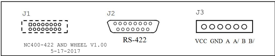
Рисунок 6.4 – Расположение разъемов платы переключателей СП NC400-7
