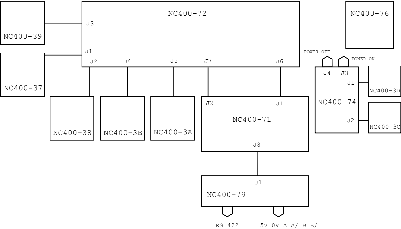
Рисунок 6.1 - Схема соединений и состав СП NC400-7
