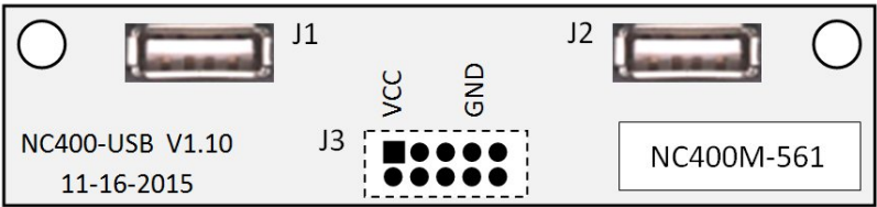
Рисунок 4.47 - Расположение разъемов платы NC400M-561
