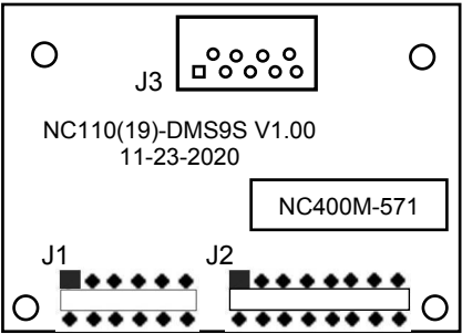
Рисунок 4.46 - Расположение разъемов платы KEY NC400M-571
