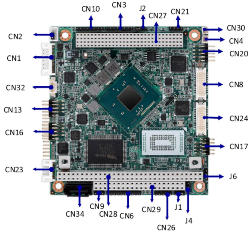
Верхняя сторона платы CPU PCM-3365
