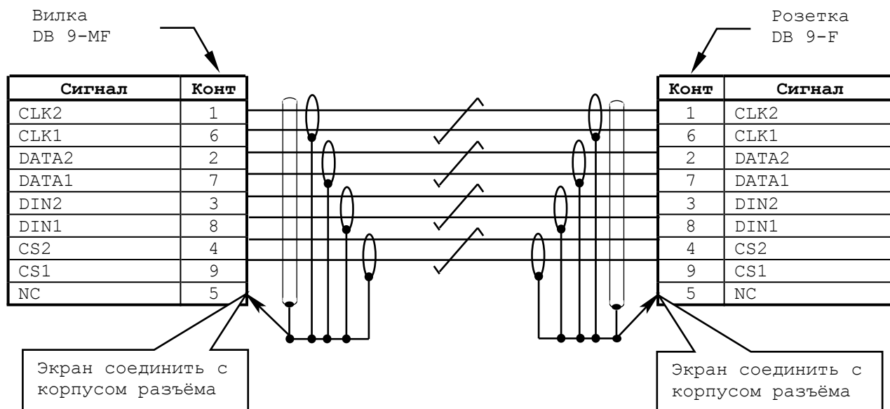
Рисунок 4.36 – Электрическая схема кабеля канала SSB NC310-81
