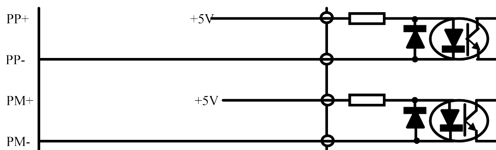
Рисунок 5.31 – Принципиальная схема подключения привода двигателя к входной линии фотоэлектрической связи
