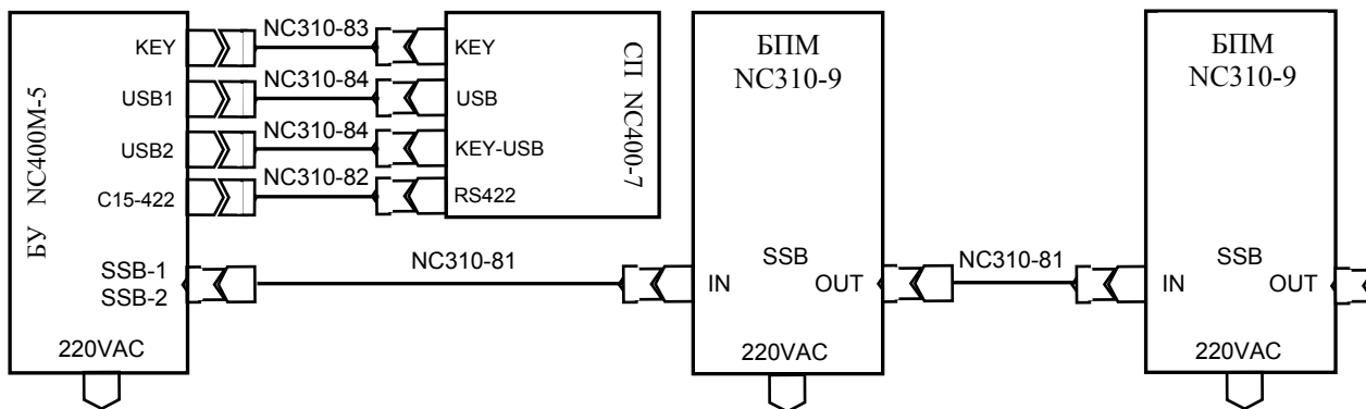
Рисунок 3.6 – Схема соединения УЧПУ NC-400М
