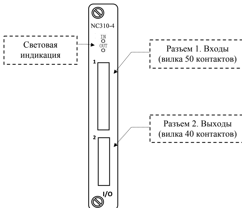
Рисунок 5.31 – Лицевая панель модуля NC310-4 (I/O)
