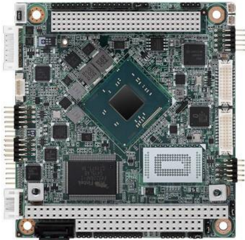
Рисунок 4.3 – Внешний вид платы CPU PCM-3365
