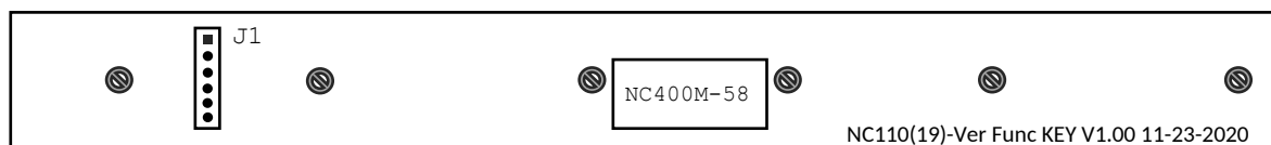
Рисунок 4.45 – Плата ФК NC400M-58, где J1 – связь с платой NC400M-571 ( J1 )
