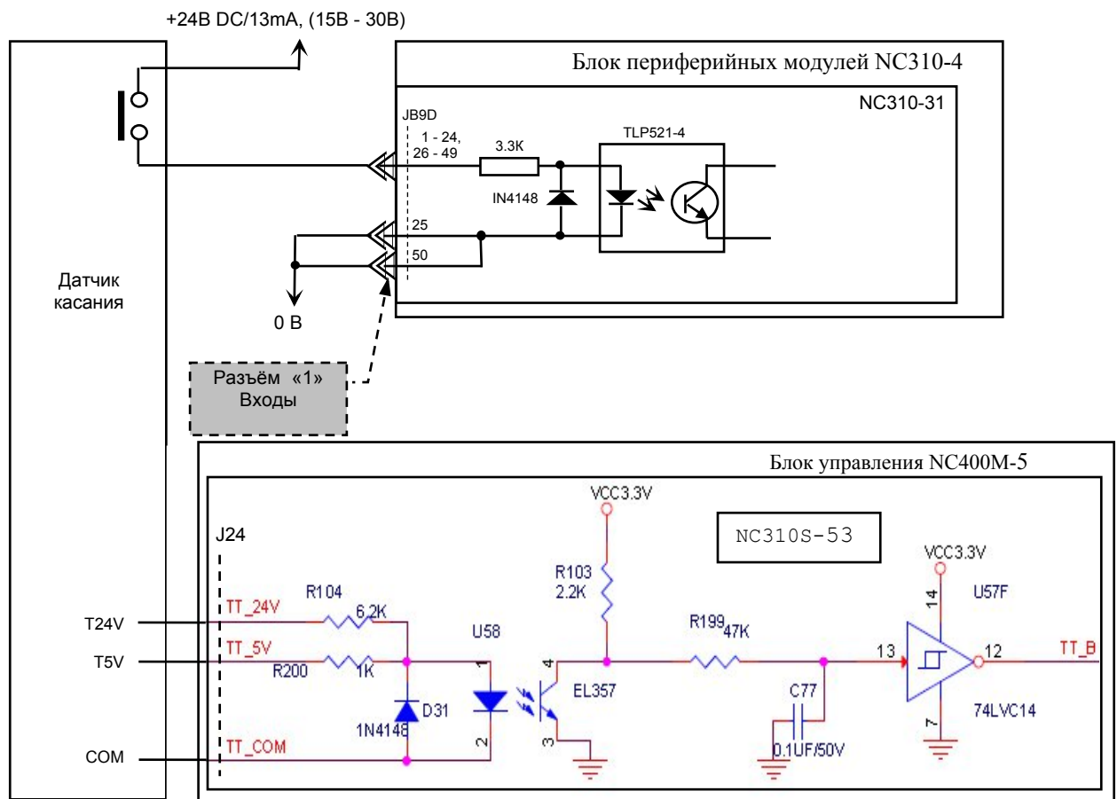
Рисунок 4.32 - Подключение датчика касания к УЧПУ NC-400M
