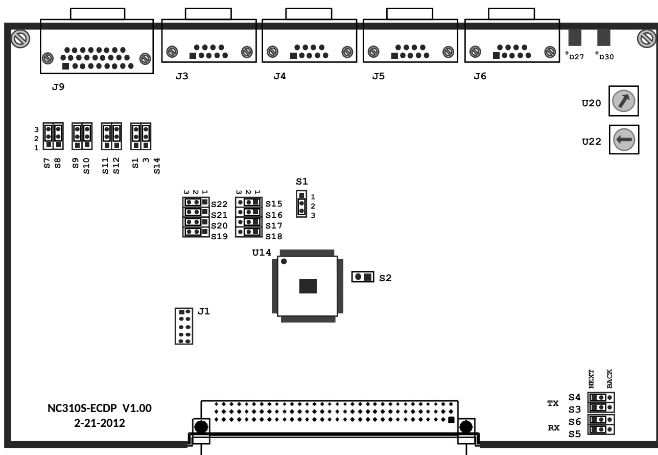
Рисунок 5.21 Расположение разъемов и перемычек модуля ЕСДР NC310-38
