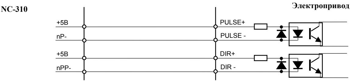
Рисунок 5.27 – Подключение дифференциальных сигналов ЦИП
