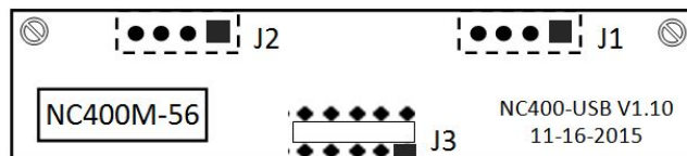
Рисунок 4.38 – Расположение разъемов платы NC400M-56
