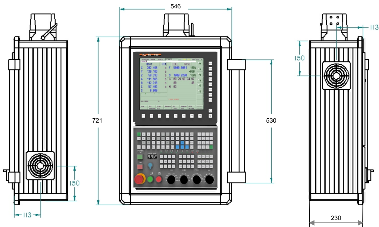
Рисунок Д.1 – Габаритные размеры кожуха для УЧПУ NC-400S.
