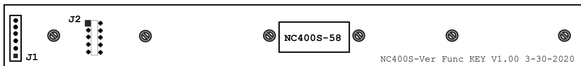
Рисунок 4.42 – Расположение разъемов платы ФК NC400S-58
