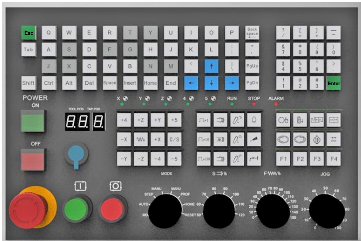
Лицевая панель станочного пульта NC400S-7
