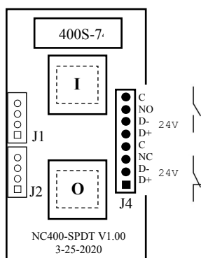
Рисунок 6.3 – Расположение разъемов платы клавиатуры СП NC400S-72 и внешнего разъема канала USB
