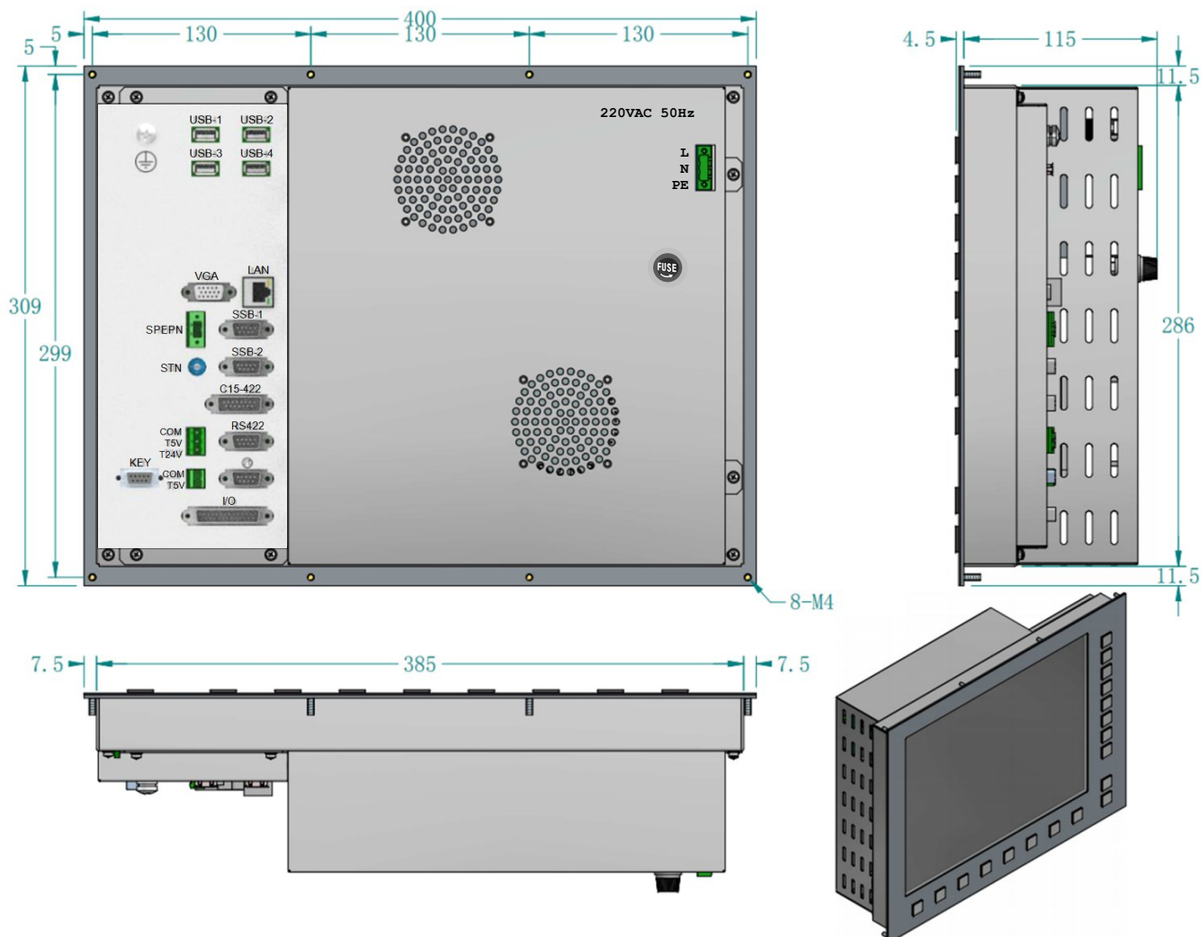
Рисунок 3.3 – Габаритные и установочные размеры блока управления NC400S-5
