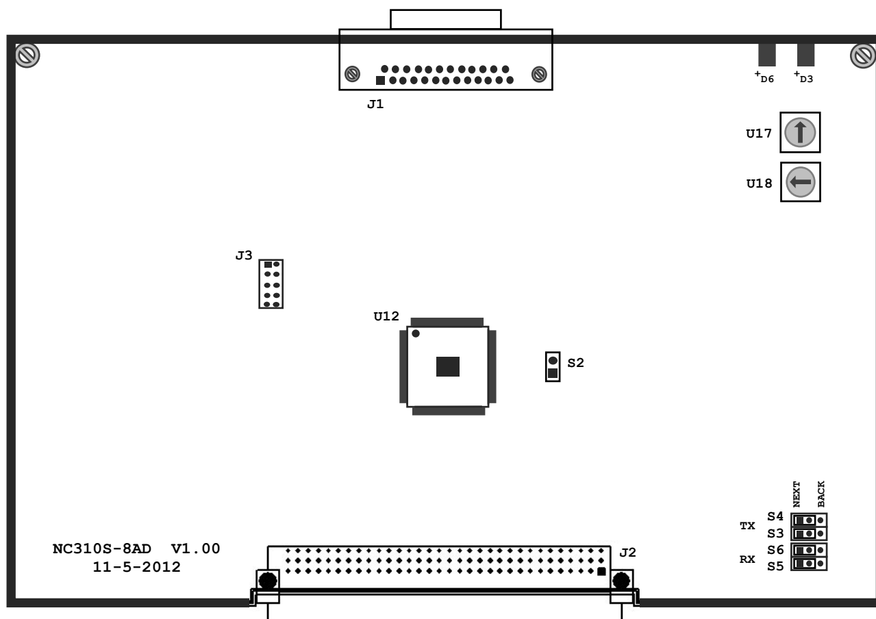
Рисунок 5.16 – Расположение разъемов и перемычек модуля A/D
