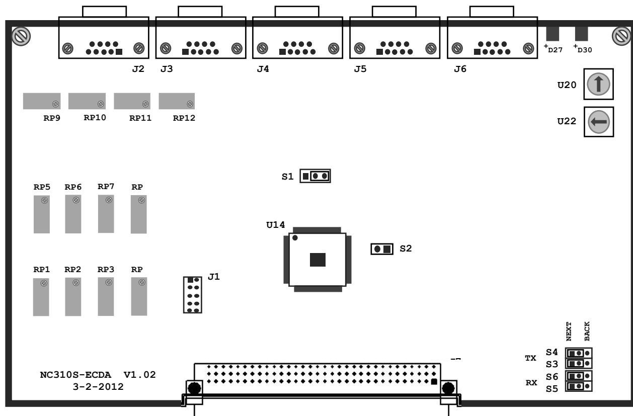
Рисунок 5.4 – Расположение разъемов и перемычек модуля ECDA
