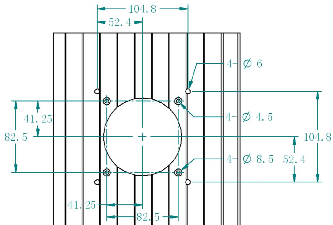
Рисунок Д.4 - Схема отверстий для монтажа системного вентилятора.
