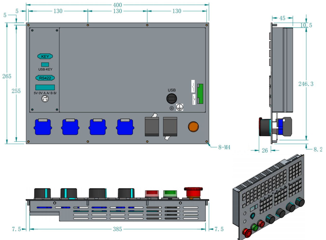
Рисунок 3.4 - Станочный пульт NC400S-7
