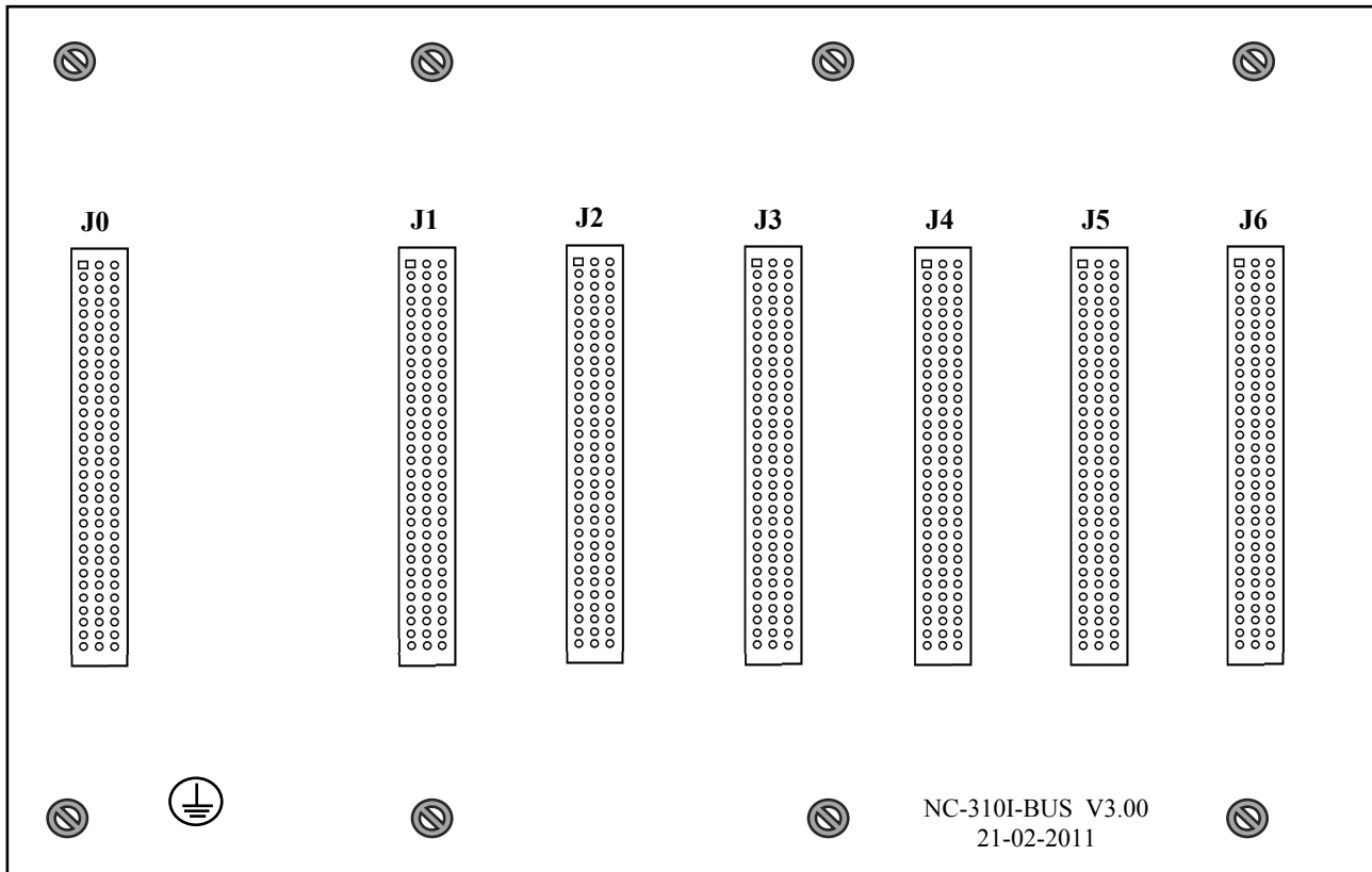
Рисунок 5.35 - Расположение разъемов модуля шины NC310-91
