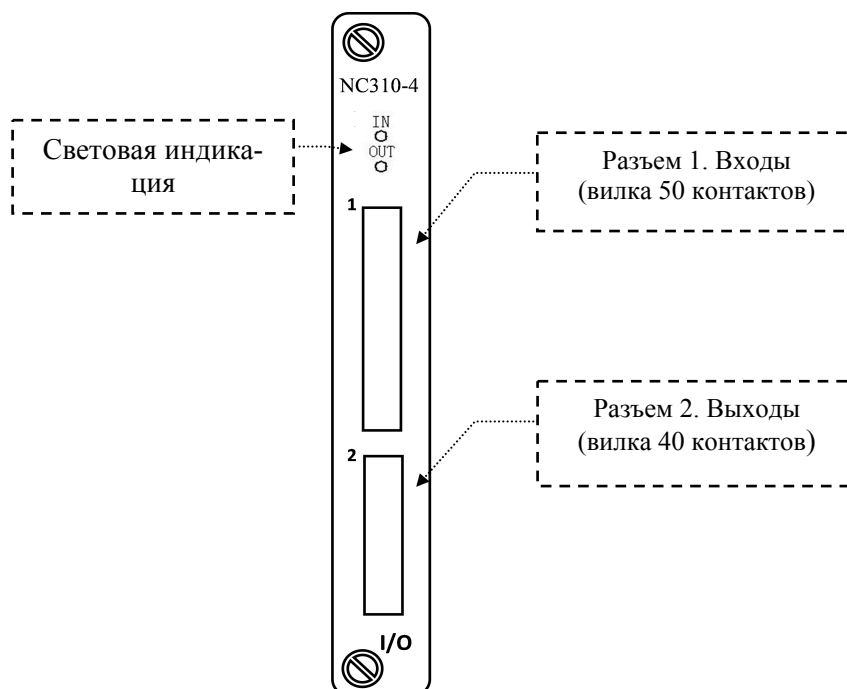
Рисунок 5.31 – Лицевая панель модуля NC310-4 (I/O)
