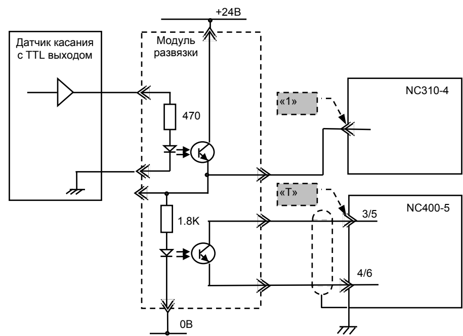
Рисунок 4.33 – Подключение датчика касания с НРК
